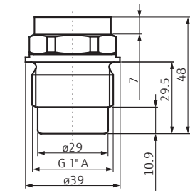
Gewinde ISO 228 G 1" Dichtung O-Ring
